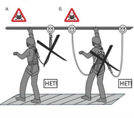
Рис. 10. Ограничения по использованию
