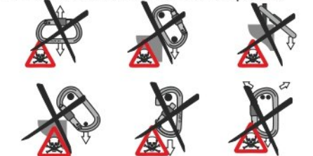
Рис. 4. Опасные способы использования карабинов
