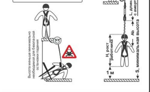
Рис. 11. Расчет высоты свободного пространства под пользователем для безопасной остановки падения
