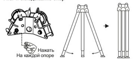
Рис. 5. Регулировка высоты
