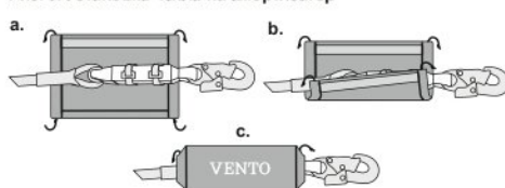
Рис. 3. Установка чехла на амортизатор
