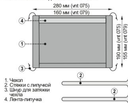
Рис. 1. Внешний вид и составные части
