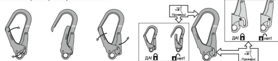
Рис. 3. Открытие / закрытие самозакрывающегося запорного элемента с фиксатором закрытого положения
