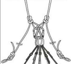
Рис. 5. Способы крепления
