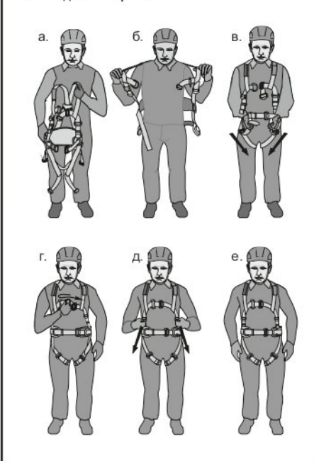
Рис. 9. Натяжение лямок
