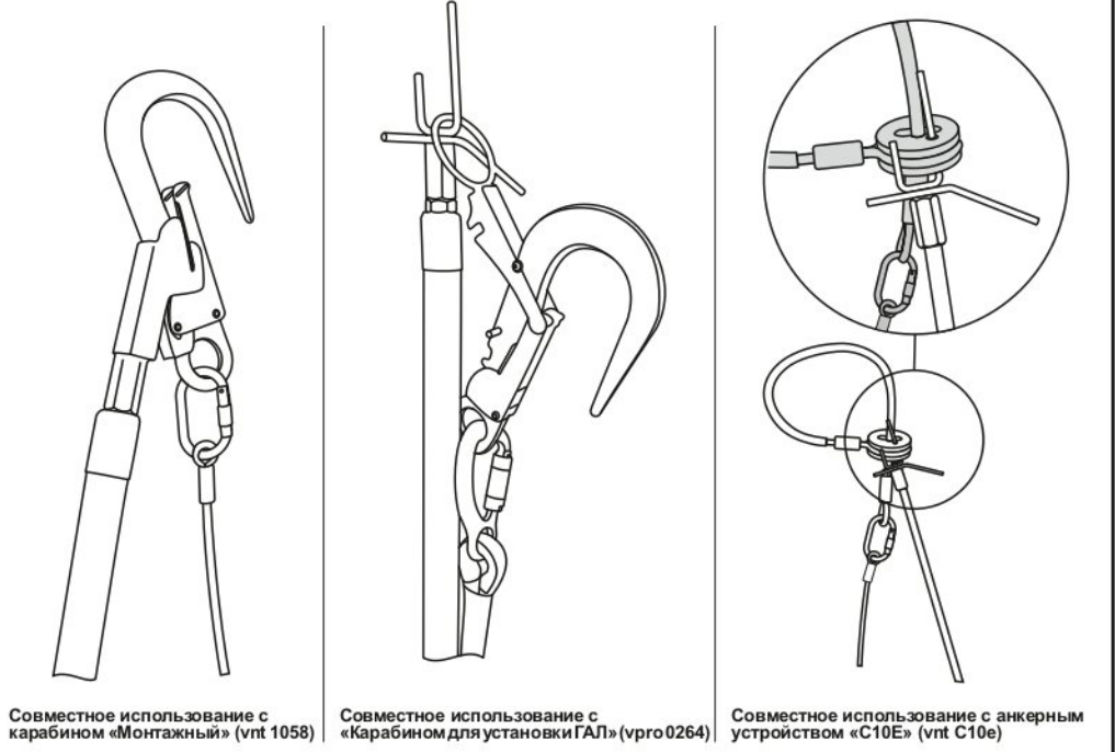
Рис. 4. Примеры использования наконечников с различными анкерными устройствами
