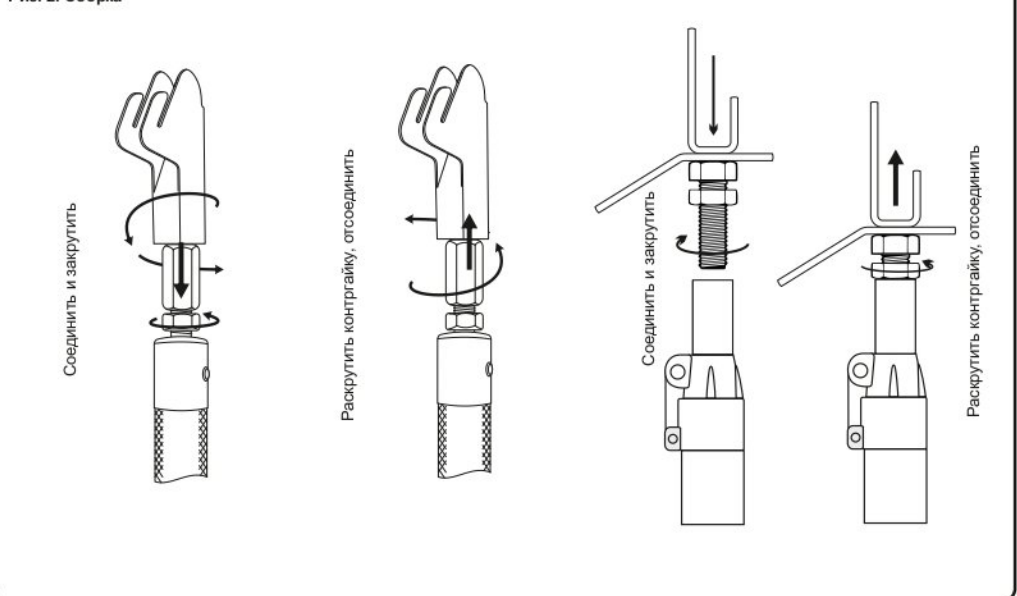
Рис. 3. Последовательность установки страховочной системы
