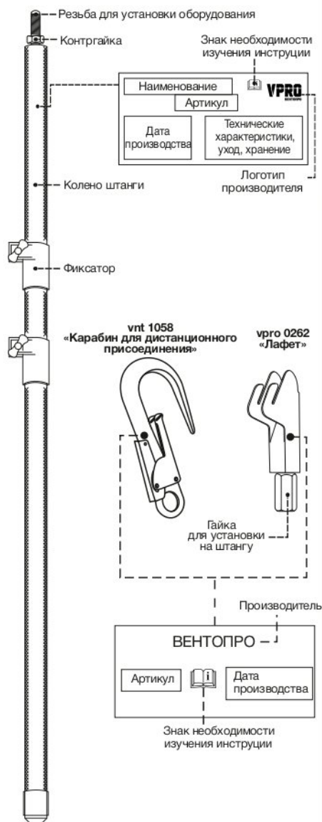
Рис. 4. Примеры использования с устройствами спасения и эвакуации
