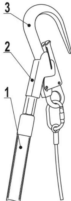
Рис. 3. Совместное использование с карабином vnt 1058
